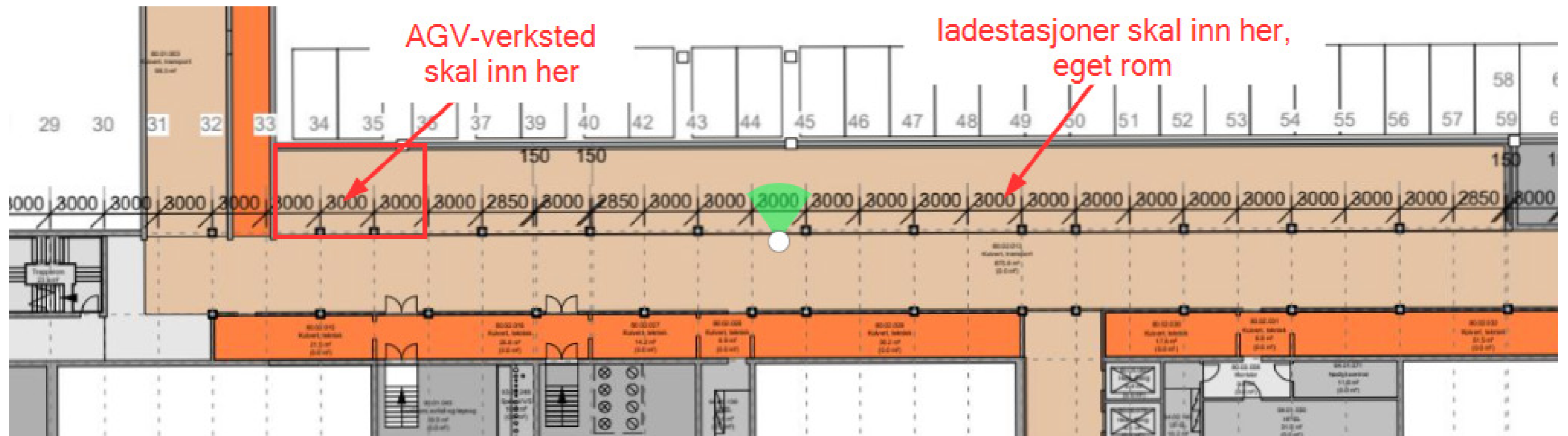
AGV ladestasjoner + verksted plasseret i kulvert / skisseforslag
